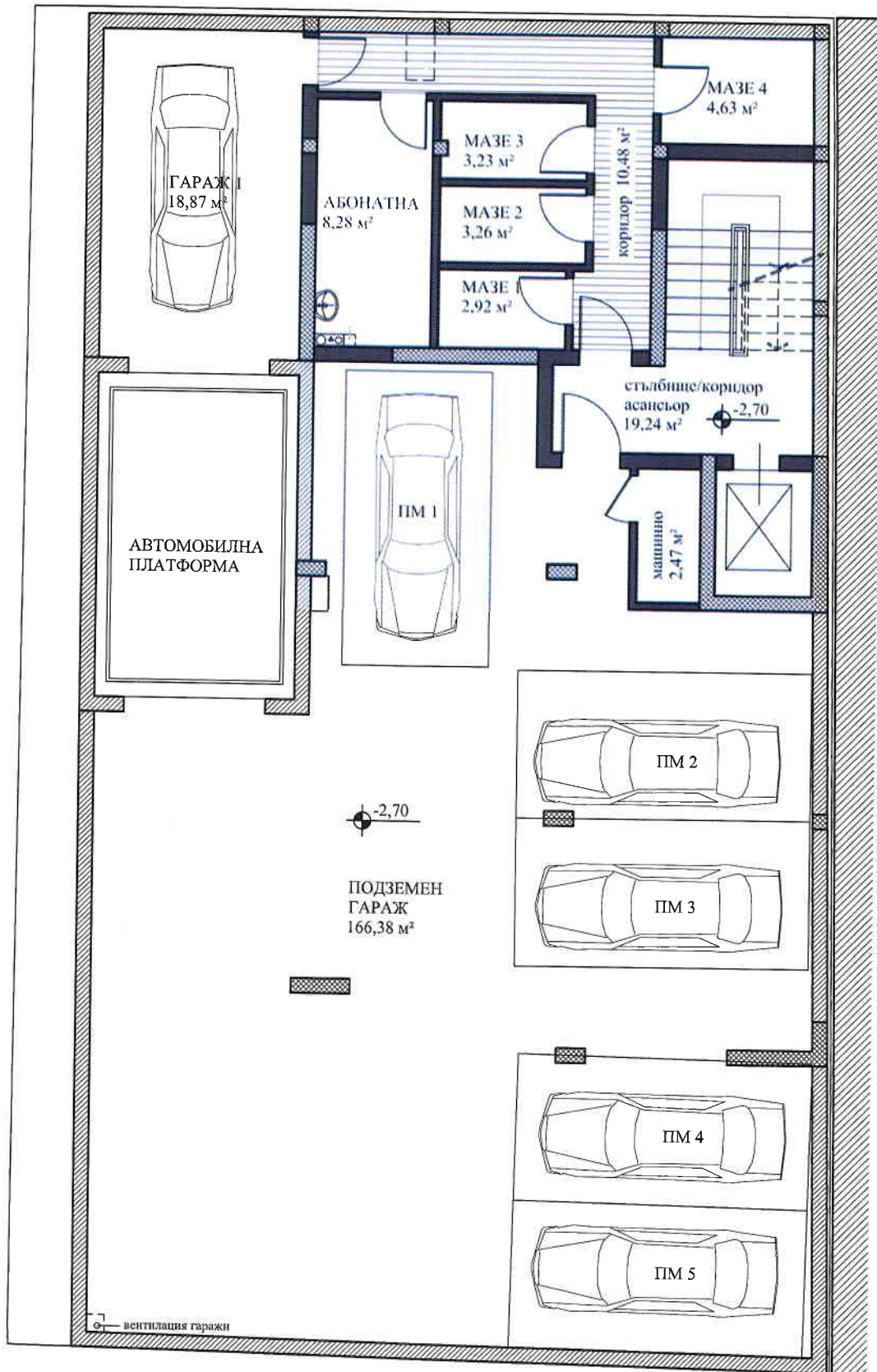
СУТЕРЕН кота - 2,70
