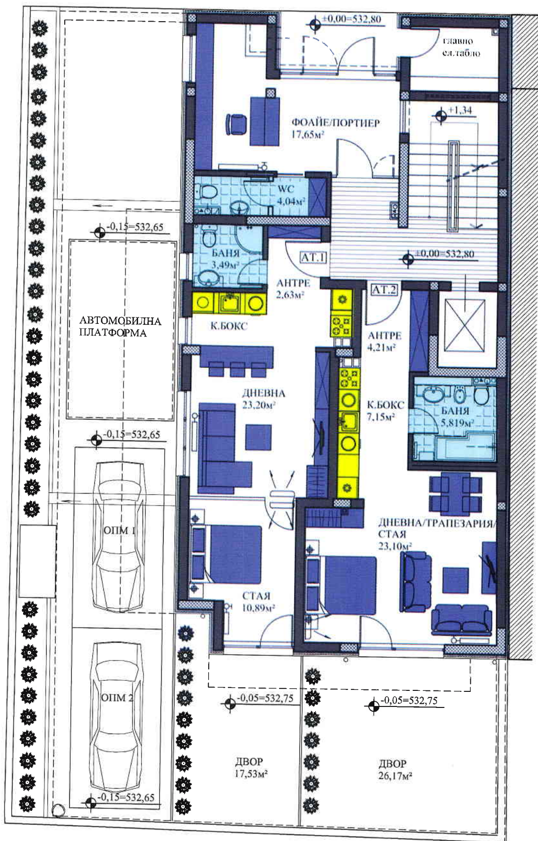
ПЪРВИ ЕТАЖ кота ± 0,00
